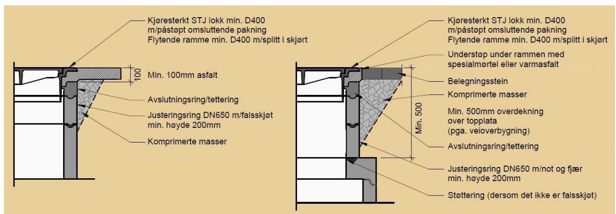
Figur 23: Viser asfaltering rundt kumlokk
