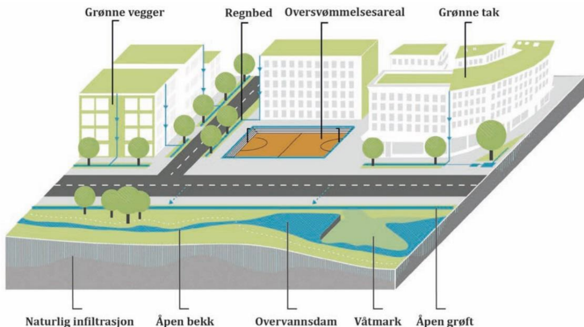
Figur 4 Lokal overvannshåndtering med ulike typer løsninger (NOU 2015:16 Overvann i byer og tettsteder)
